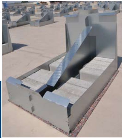
Beschwerung mit Kies oder Formsteine
